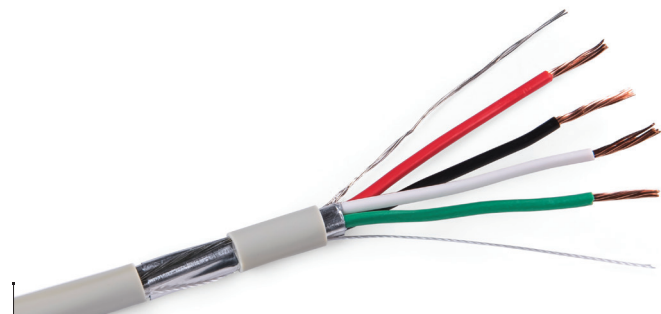
Multiconducteur 18 AWG blindé, 4 conducteurs, 18 brins Disponible en: 500 pi (boîte)/1000 pi (rouleau), riser et plénum Produit no. 18AWG-4C-STR-SH-QQQ-XX-YYYY
