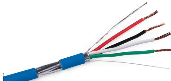
Multiconducteur 22 AWG blindé, 4 conducteurs, 7 brins Disponible en: 500 pi (boîte)/1000 pi (rouleau), riser et plénum Produit no. 22AWG-4C-STR-SH-QQQ-XX-YYYY
