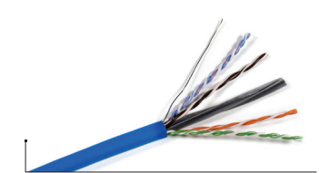
Paire de 4 riser solide Cat 6A Disponible en plénum et riser Produit no. UTP4-C6A-SOLID-CMR-BL-305
