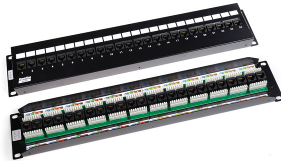
24 ports Cat 5e, type 110 Disponible en 12 et 24 ports Produit no. PPW1-24-8P8C-C5E-FR
