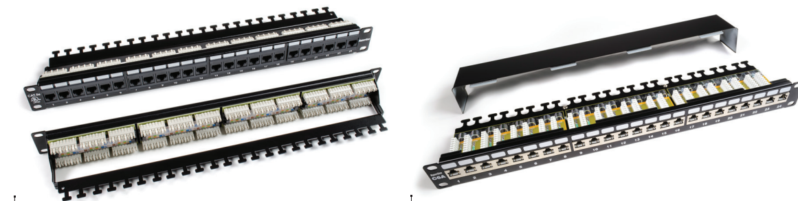
24 ports Cat 5e, type 110 Disponible en Cat 5e et Cat 6, en 24 et 48 ports. Gestionnaire arrière vendu séparément Produit no. PP3-19-24-8P8C-C5E-110
