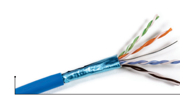
Paire de 4 plénum blindé Cat 5e Disponible en plénum et riser Produit no. FUTP4-C5E-SOLID-CMP-BL-305
