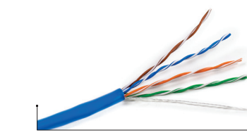
Paire de 4 riser solide Cat 5e Disponible en plénum et riser Produit no. UTP4-C5E-SOLID-CMR-BL-305
