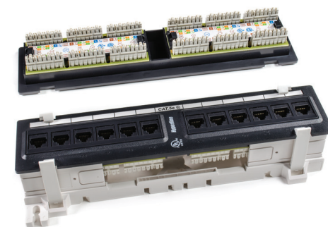
12 ports Cat 5e, type 110 Disponible en Cat 5e et Cat 6 Produit no. PPW1-12-8P8C-C5E
