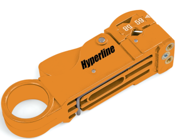
Dénudeur de câble coaxial pour RG58 et RG59
