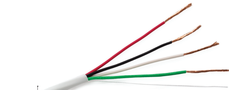
Câble haut-parleur 16/4, 65 brins, riser Disponible en boîte (dévidoir) de 500 pi Produit no. SPK4-16AWG-CU9-STR-CMR-XX-500F
