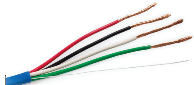
Câble haut-parleur 14/4, 105 brins, riser Disponible en boîte (dévidoir) de 500 pi Produit no. SPK4-14AWG-CU9-STR-CMR-XX-500F
