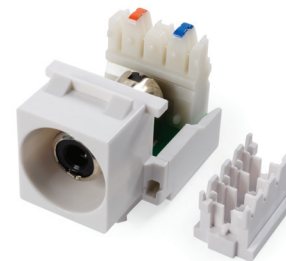
Connecteur Keystone pour RCA – 110 Produit no. KJZZ***1-RCA-110-XX*
